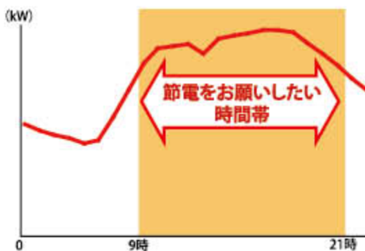
■冬の平日の電気の使われ方 (昨冬ピーク発生日 平成23年2月14日)
