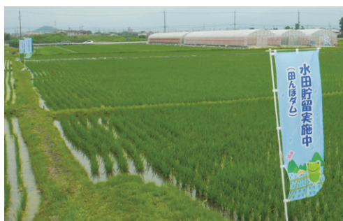
水田を活用した貯留対策(田原本町)
