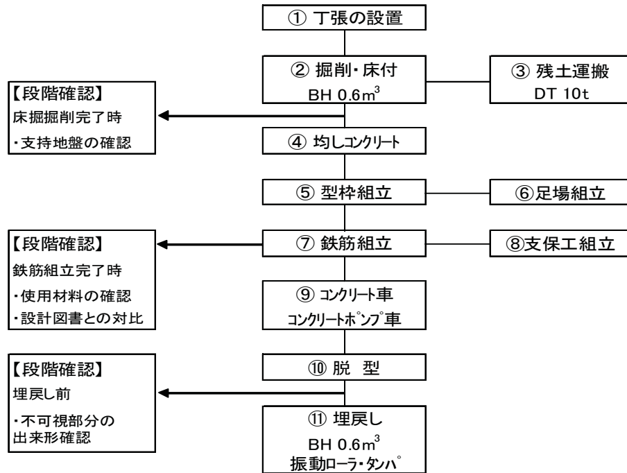
[作業フロー(重力式擁壁)の記載例]
