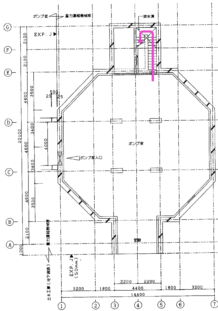
地下1階平面図
