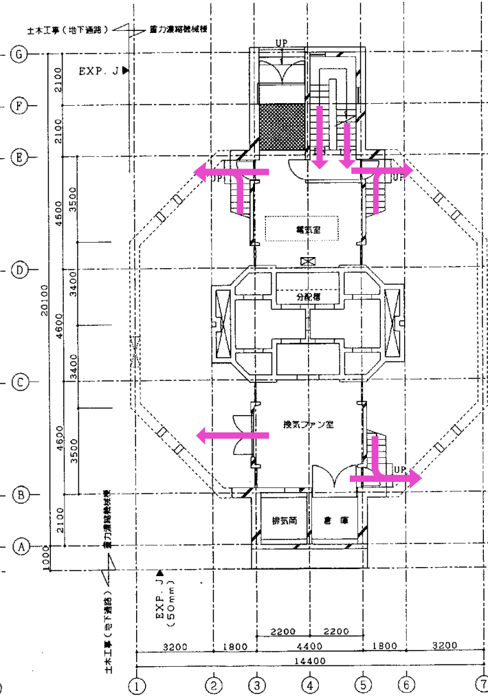
1階平面図 (避難階)
