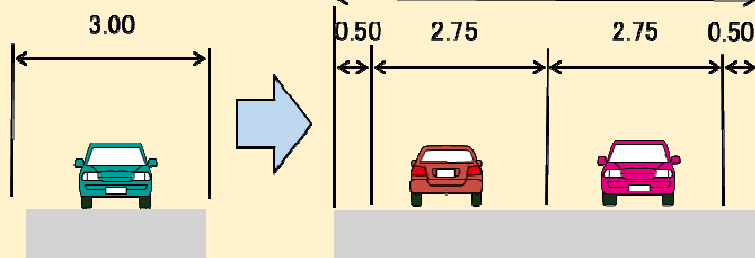
◆標準断面図
