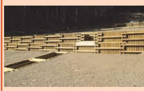
間伐材二重井桁枠工 (間伐材)
