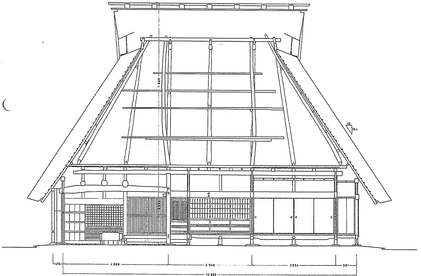
第7図 竣工 梁間断面図 1:100
