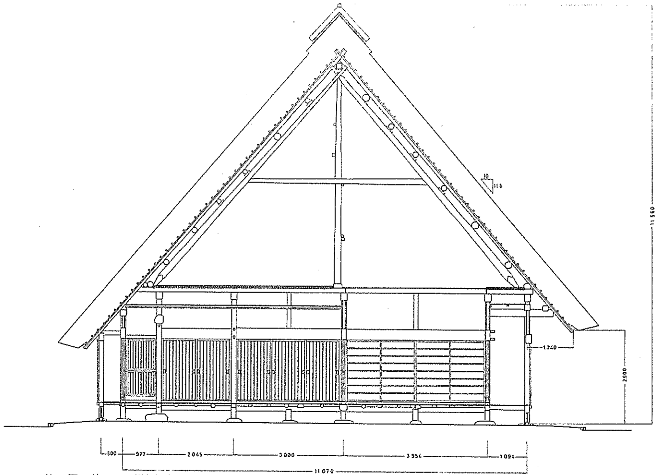
第7図 竣工 梁間断面図 1:100
