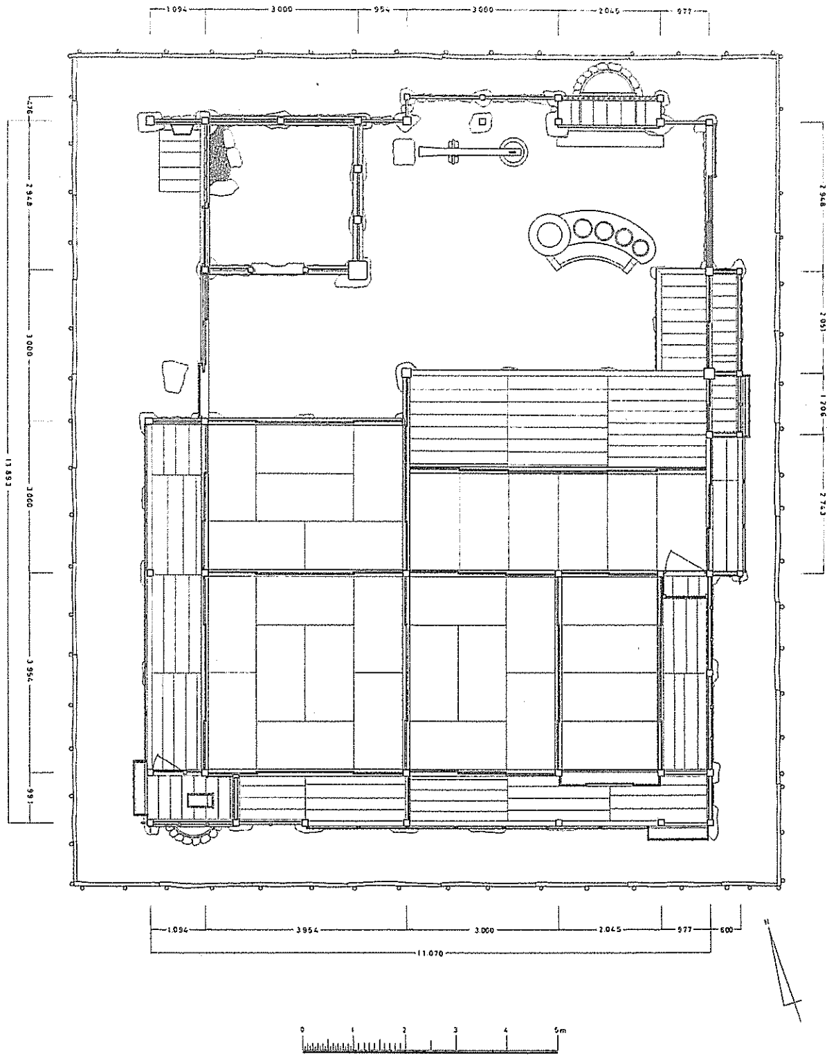
第1圖 竣工 平面圖 1:100
