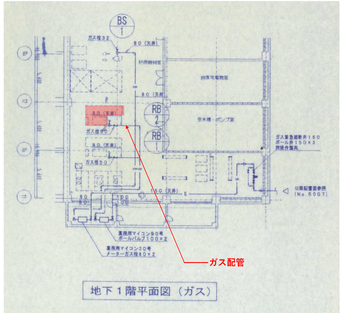
ガス配管図
