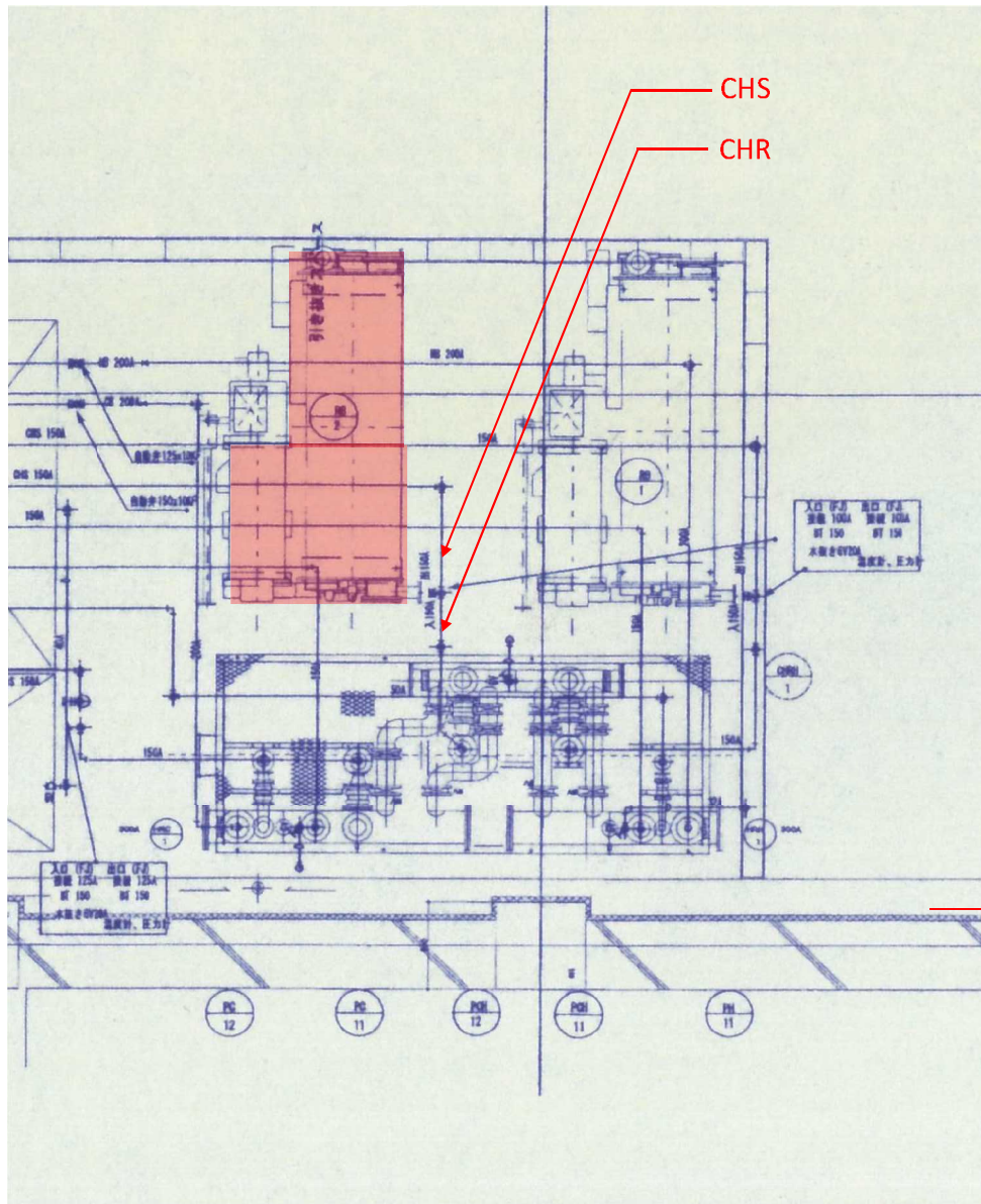
冷温水配管図
