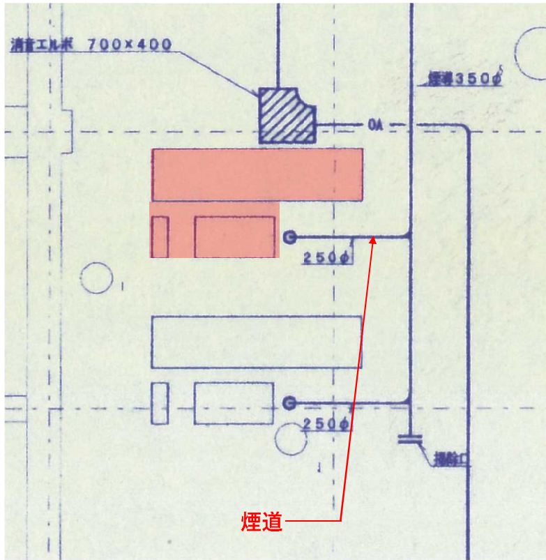
煙道配管図
