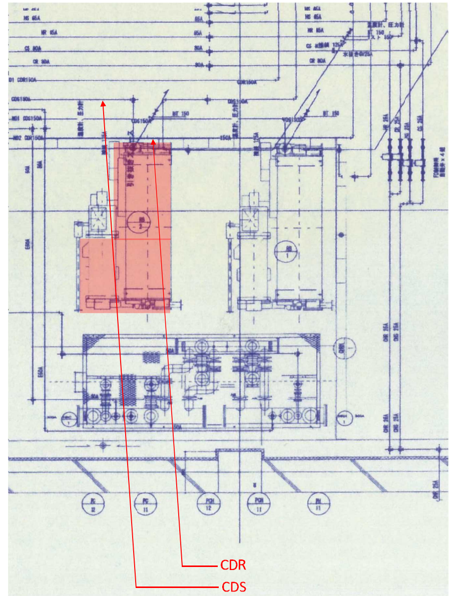
冷却水配管図
