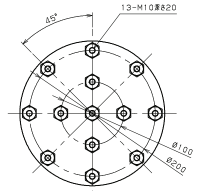
可動部パターン (尺度: 1/3)
