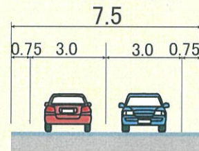
◆ 標準断面図
