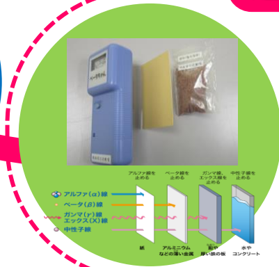
ベータ線測定実験
