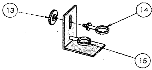
眼球固定器
