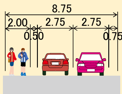
◆標準断面図
