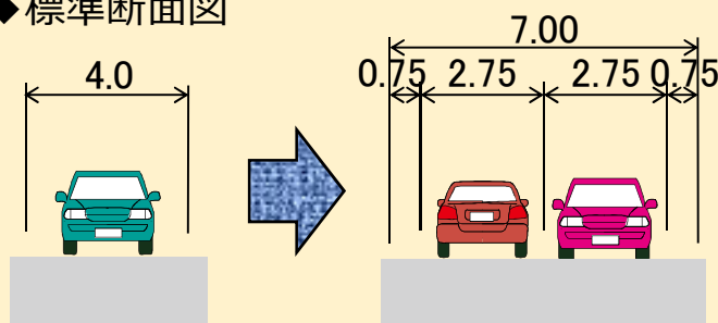
◆標準断面図
