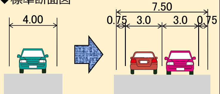
◆標準断面図
