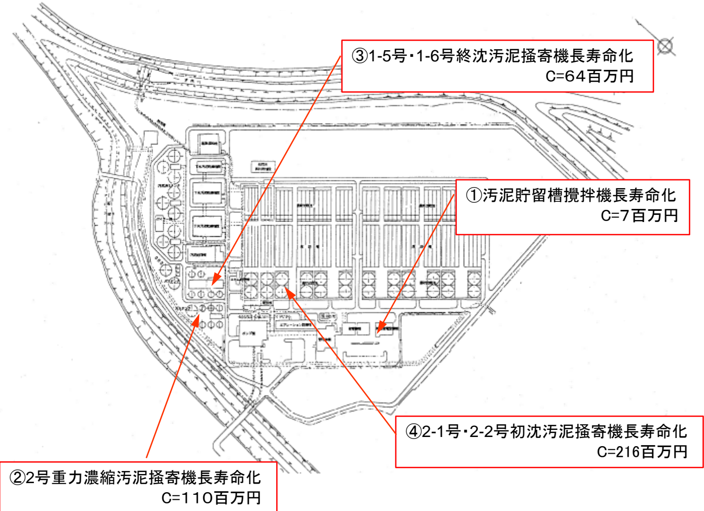
第二浄化センター平面図
