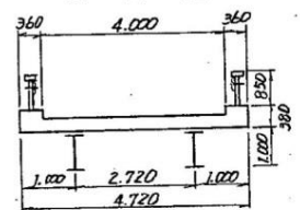
断面図
