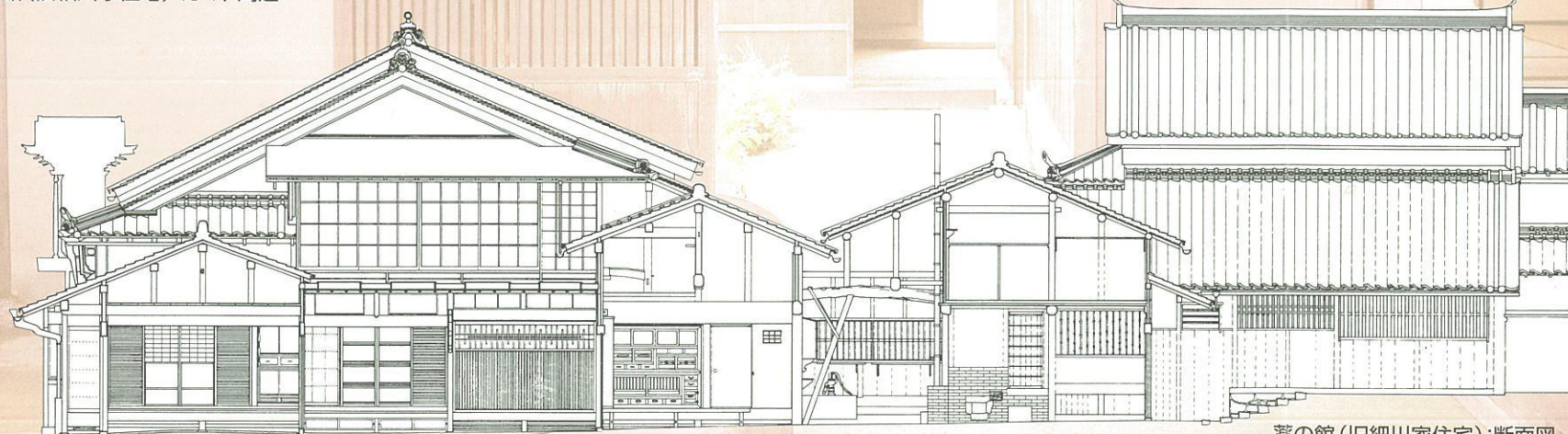
薬の館(旧細川家住宅):断面図 東京芸術大学建築科・作成
