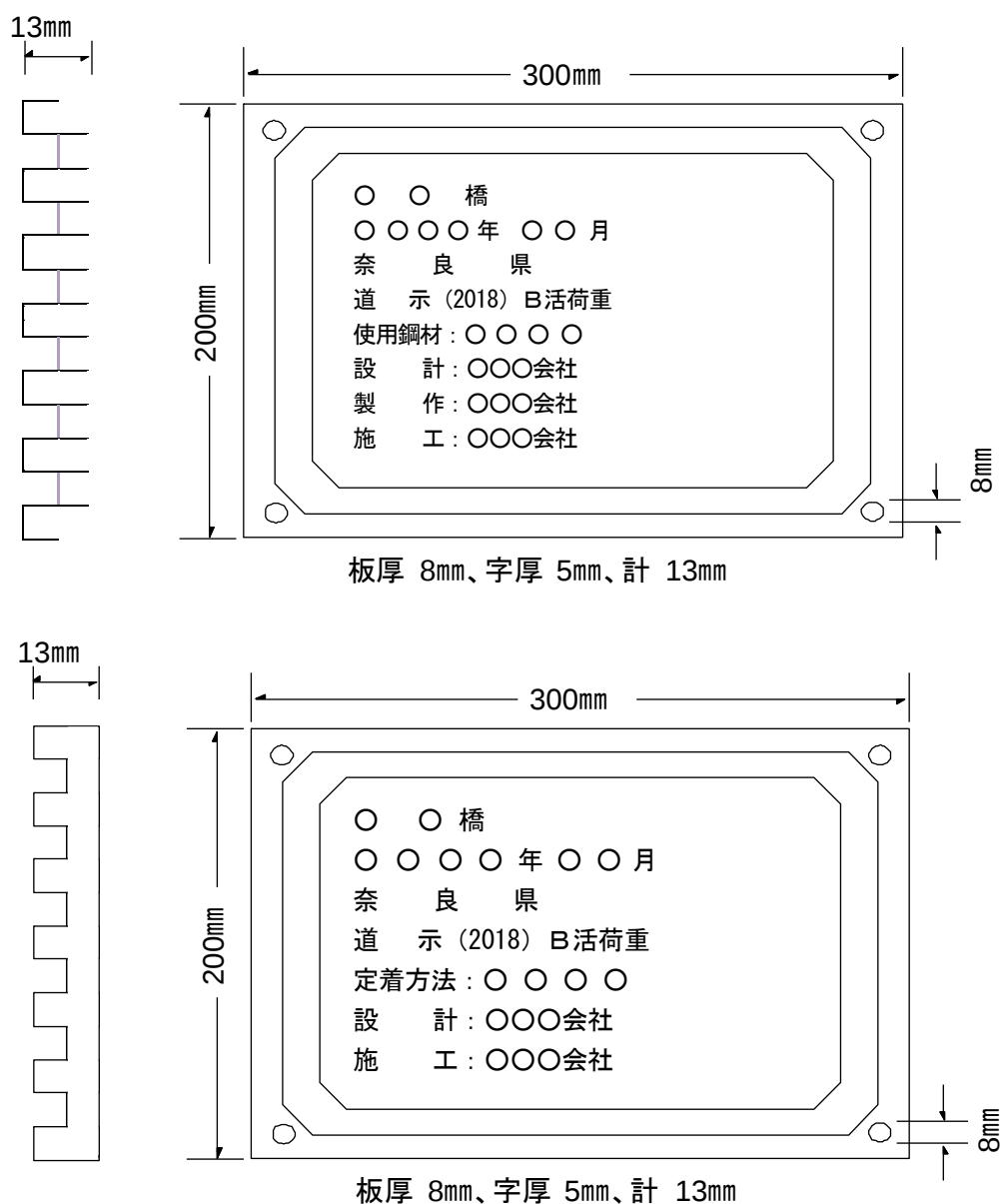
図3-2-2 銘板の寸法及び記載事項
