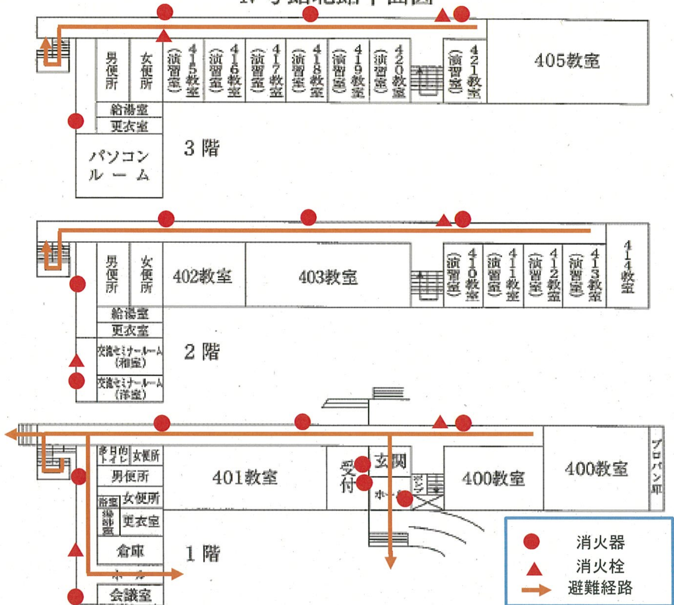
IV号館北館平面図
