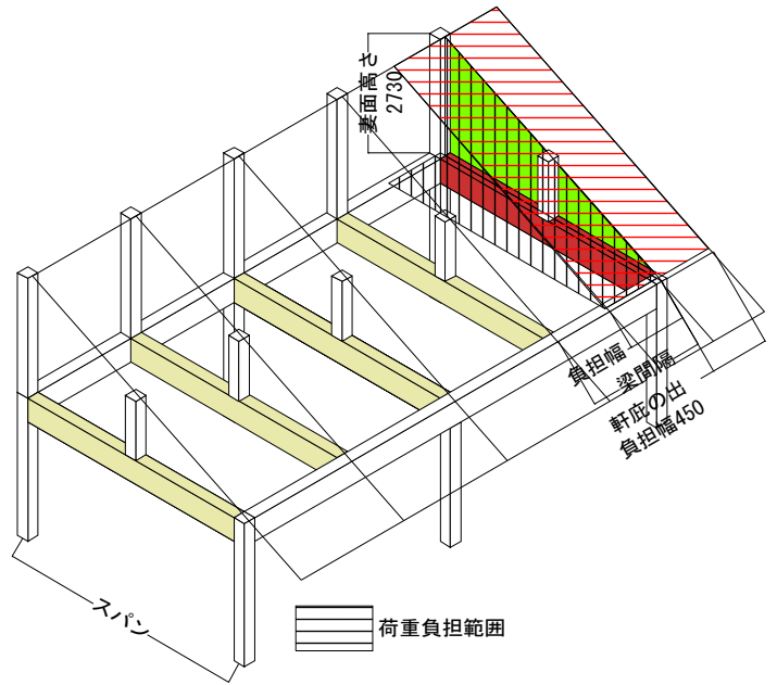
小屋組、外壁、軒庇荷重
