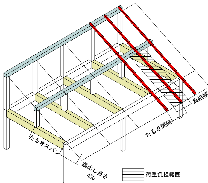
軒庇荷重
