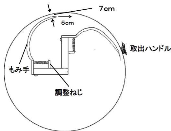
図 9 中揉機バネ圧の測定方法
