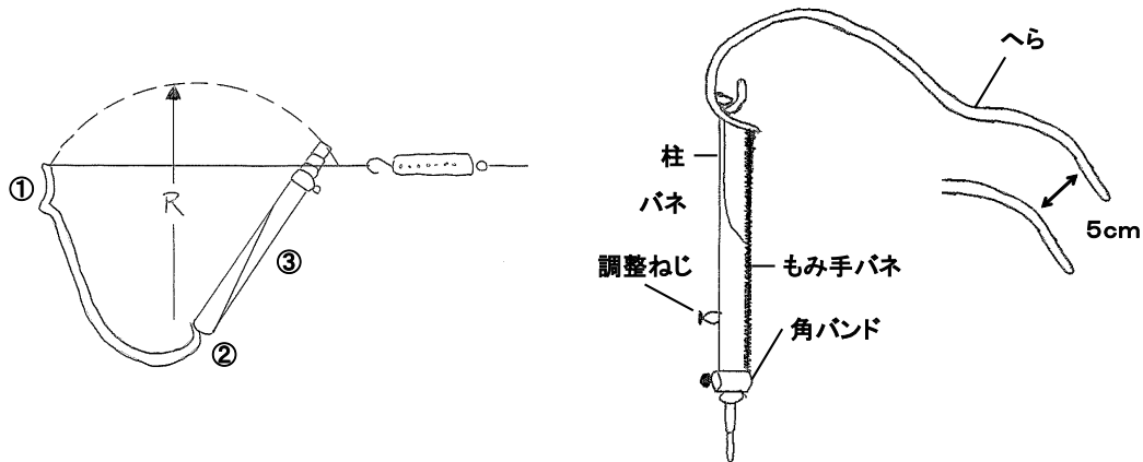
図7 もみ手のバネ圧の測定方法
