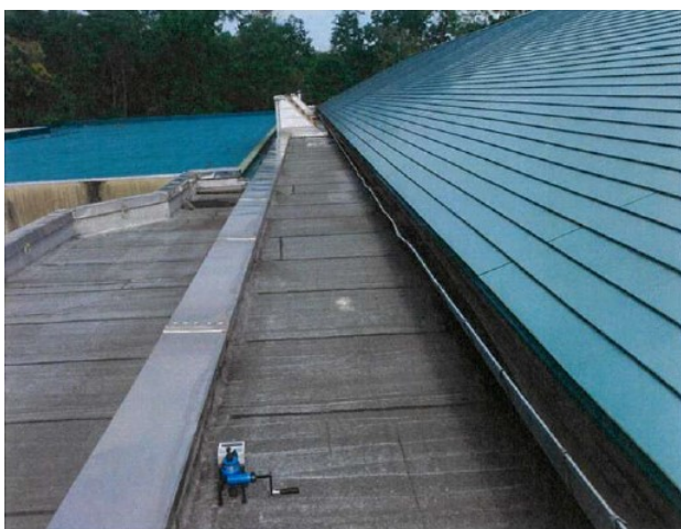
屋根（改修前）
