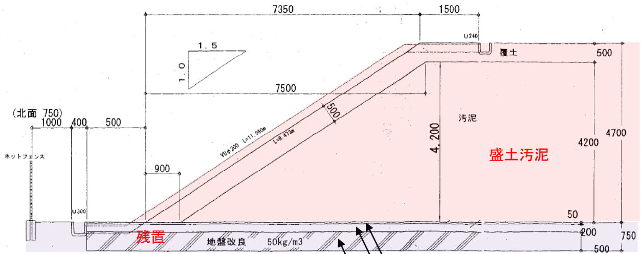
断面詳細図 1:40
