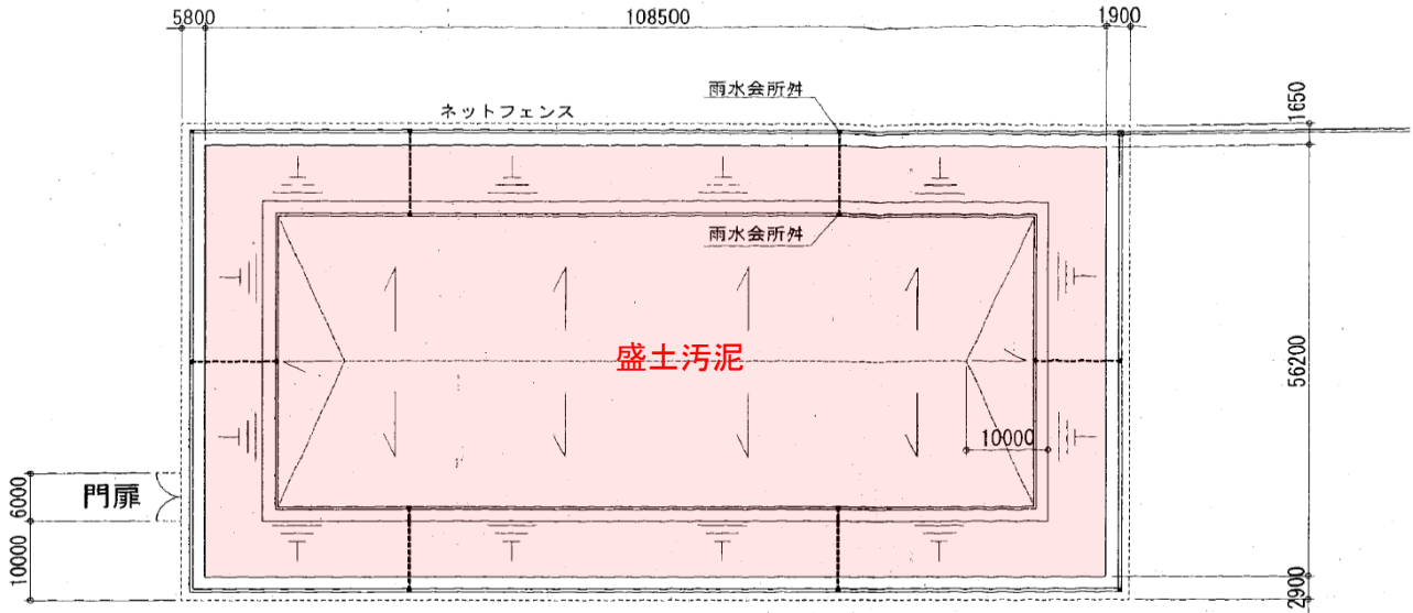
処分地平面図 1:400
