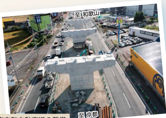
京奈和自動車道の整備 （大和北道路）
