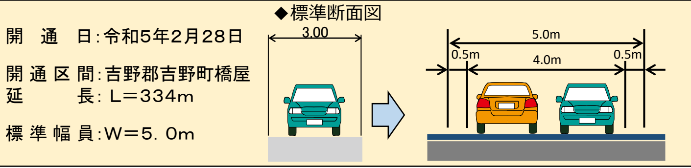
現道部
