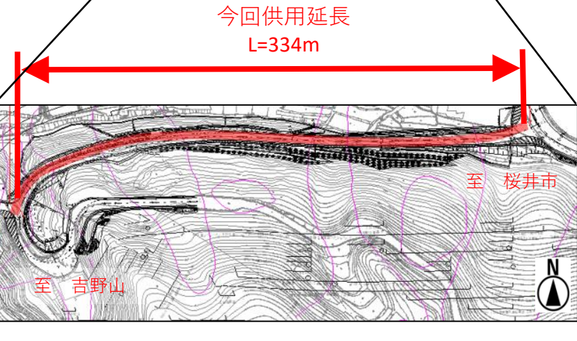
整備後
