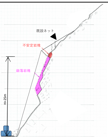
崩壊部の横断図
