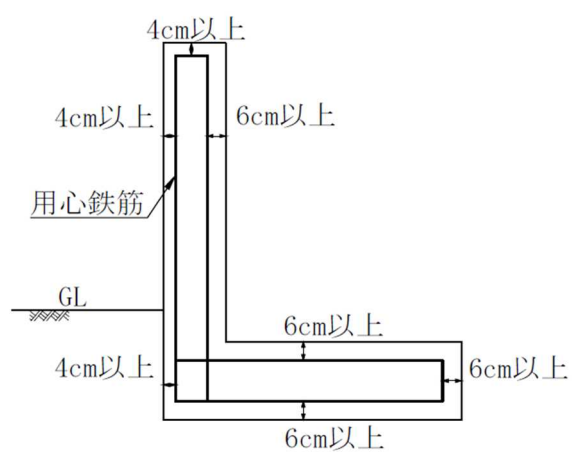
図 3-1 9 鉄筋の被り
