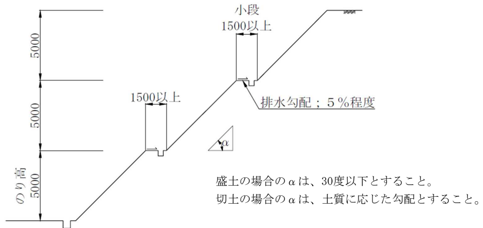
図2-1 のり面標準断面図（単位：mm）
