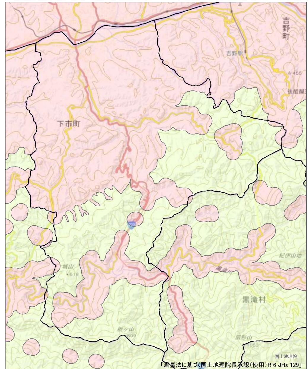
詳細位置図(S=1:57,000)
