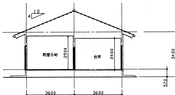
断面図
