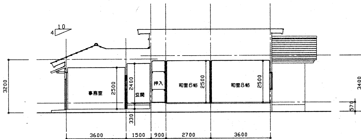
断面図
