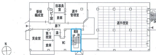
2階平面図 (S=1/300)
