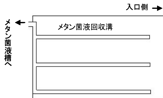
図2 発酵槽床
