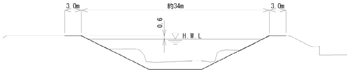
図(2)-2 新橋付近の横断面図※
