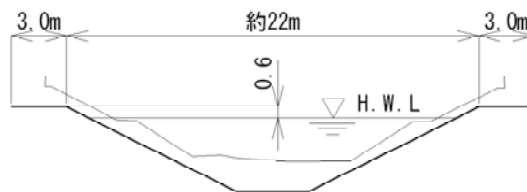
図(2)-3 金塚橋付近の横断面図※
