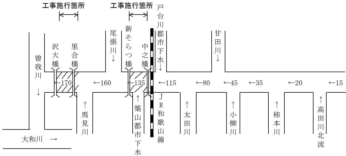
図(2)-1 計画高水流量配分図
