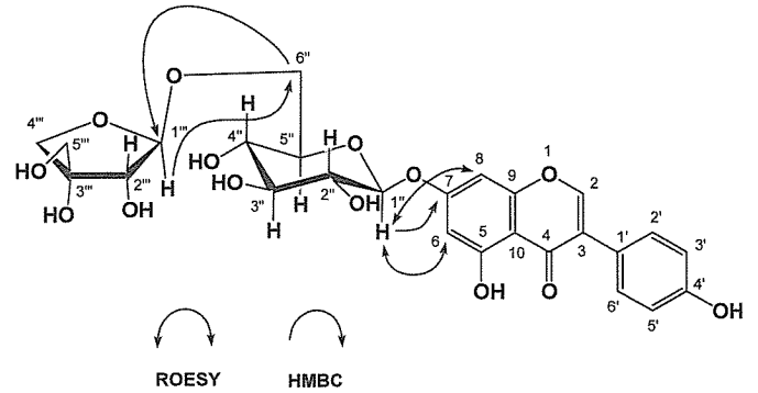
第1図 ACE阻害活性物質の構造と主要なHMBCおよびROESY相関
