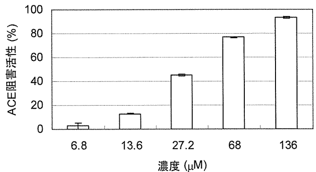
第2図 単離した ACE 阻害活性物質の活性 (平均値 \pm 標準偏差, n=3) Fig. 2. Activity of isolated ACE inhibitor (Mean \pm SD, n=3).
