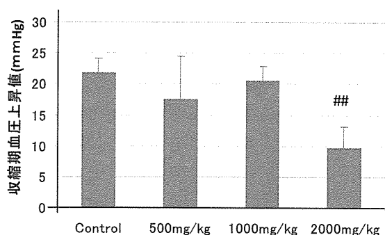
第3図 アンジオテンシン I 負荷マウスに対するクズ葉抽出物の効果 (左: 水抽出物、右: エタノール抽出物、平均値±標準誤差、n=8、##: p<0.01 vs. control)
