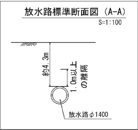
【横断面図】
