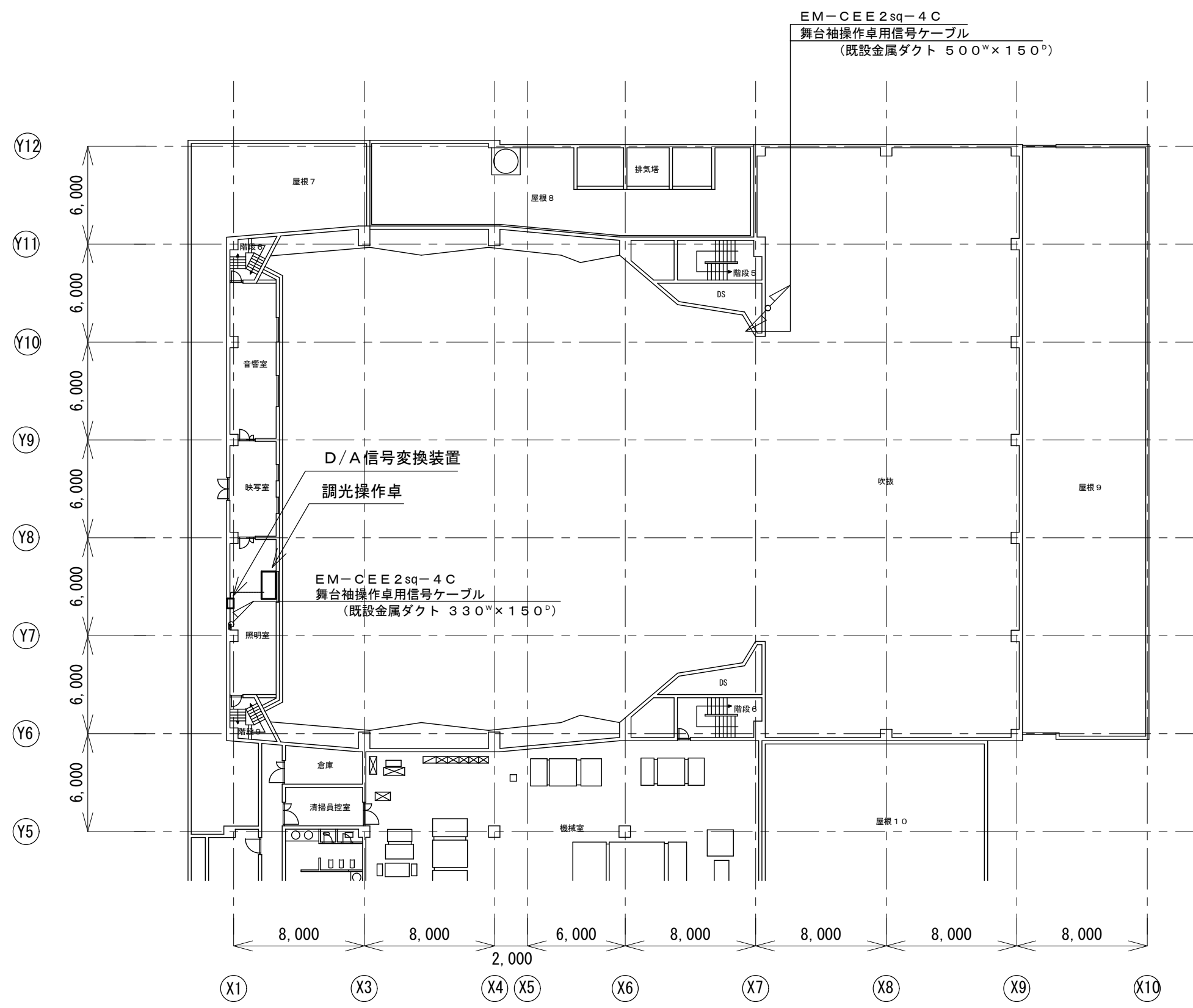
3 階平面図
