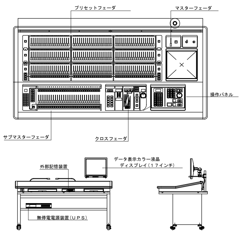
調光操作卓 S=1/20, 1/40 (参考図)
