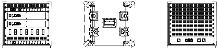
D/A信号変換装置 S=1/20 (参考図)
