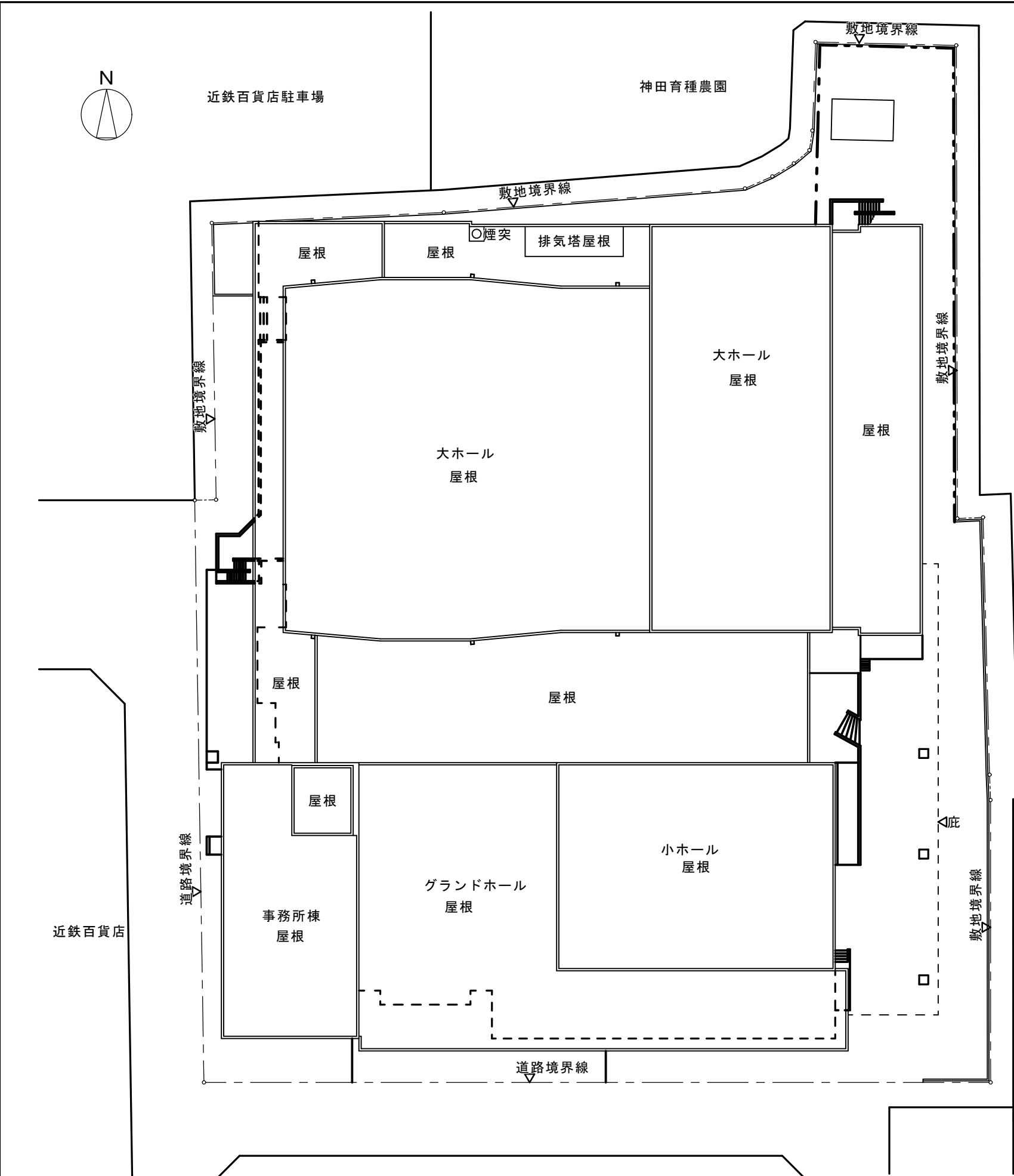
配置図 S=1/400
