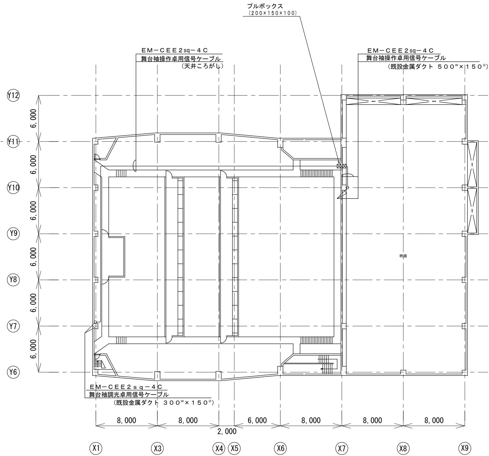
R階平面図
